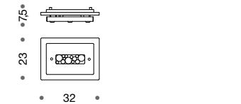
432/32 1 x G24q-2 18W CE ⊕ ▽
