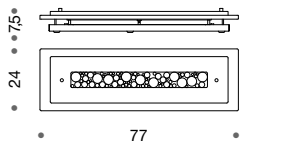
432/77 2 x FQ/T5 24W CE ⊕ ▽
