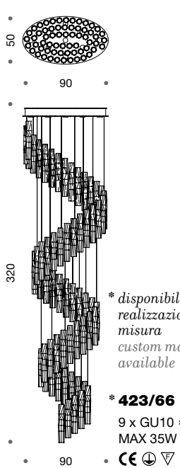
* disponibili realizzazioni su misura custom made sizes available * 423/35 6 x GU10 MAX 35W CE
