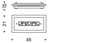
432/45 2 x G24q-2 18W CE ⊕ ▽
